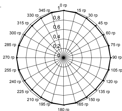
ДН в азимутальной плоскости ПЛОСКОСТИ
